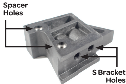
FIG. 2 TOP ASSEMBLY
